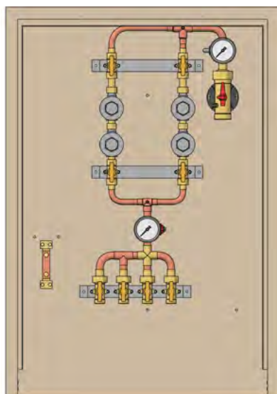
ADPV241 Armoire 1ère détente Haute Pression 40 kg
