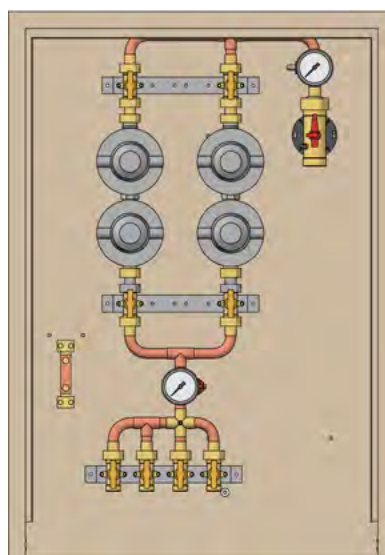
ADPV441 Armoire 1ère détente Haute Pression 150 kg
